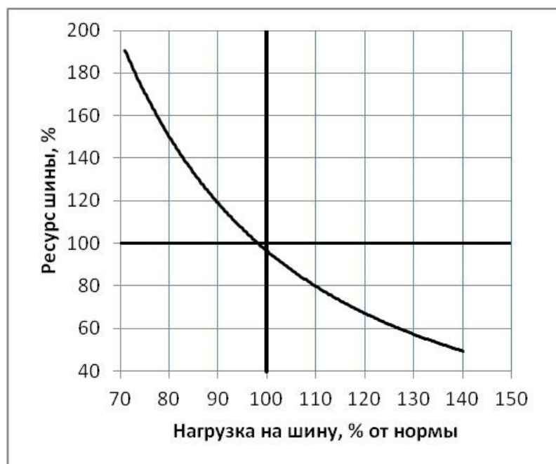
Зависимость ресурса шин от нагрузки
