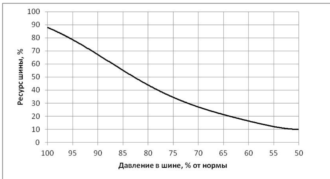
Зависимость ресурса шин от внутреннего давления
